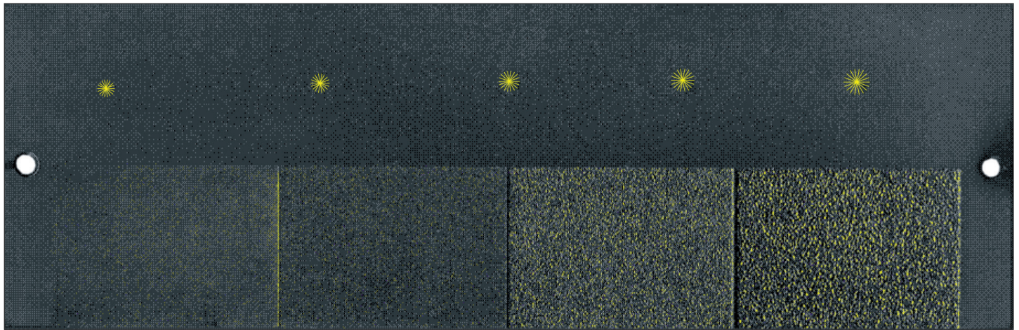
Kontrollkörper 2 nach DIN EN ISO 3452-3
